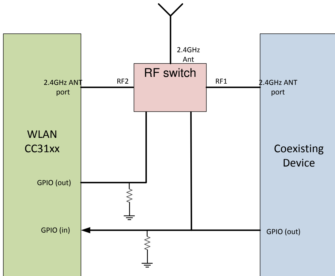
Figure 4-2. BLE Coexistence
