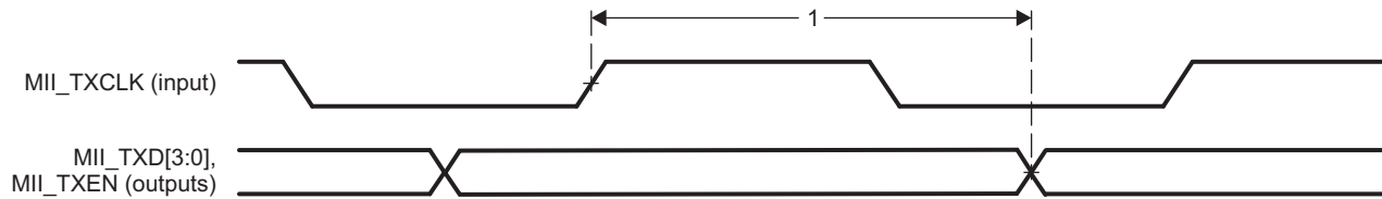
Figure 7-97. PRU-ICSS MII_TXD[3:0], MII_TXEN Timing
