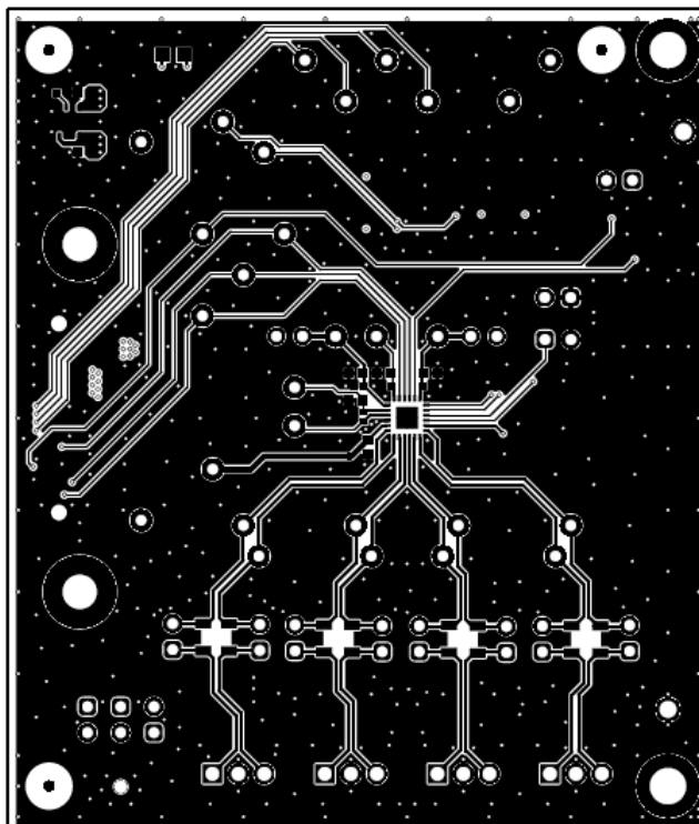
Figure 4-2. Top Layer
