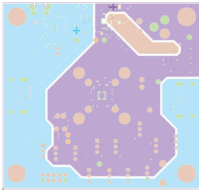
Figure 20. Layer 4 (Power)
