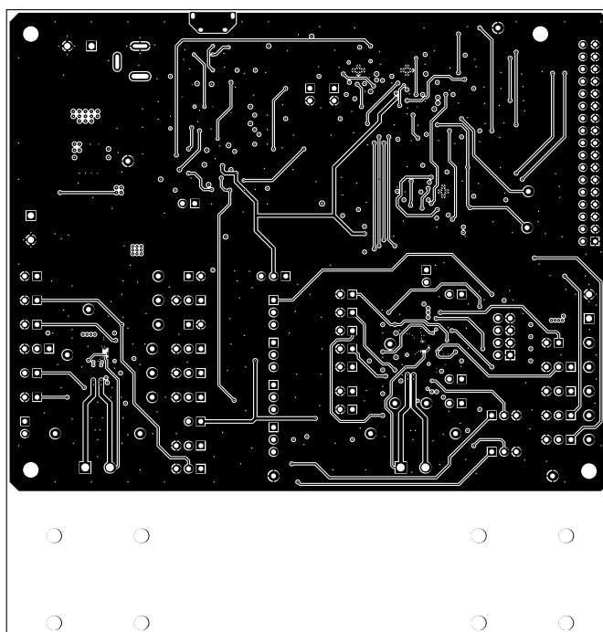
Figure 20. Bottom Layer
